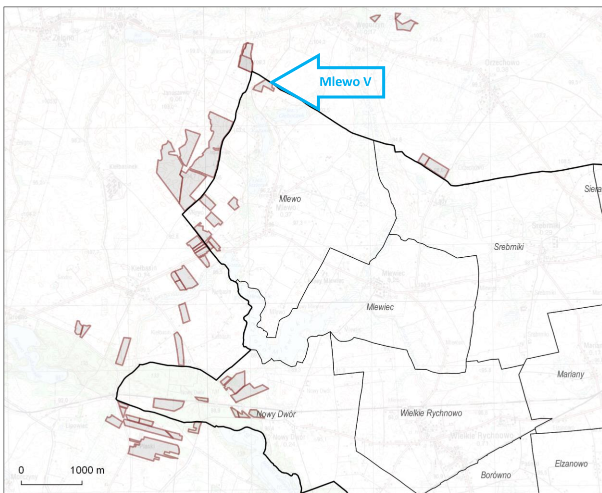
Rysunek 3. Położenie złoża „Mlewo V” na tle innych złóż (kolor brązowy) wydzielonych w obrębie szlaku sandrowego (źródło: geoport.al.gov.pl, System Gospodarki i Ochrony Bogactw Mineralnych „MIDAS”)
