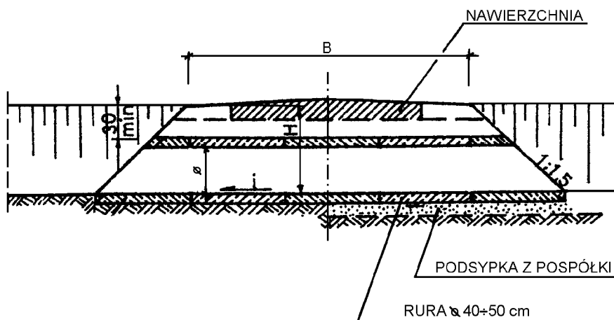
Rys. 2.1. Przekrój podłużny przepustu z rury polietylenowej średnicy 40 \pm 50 cm
